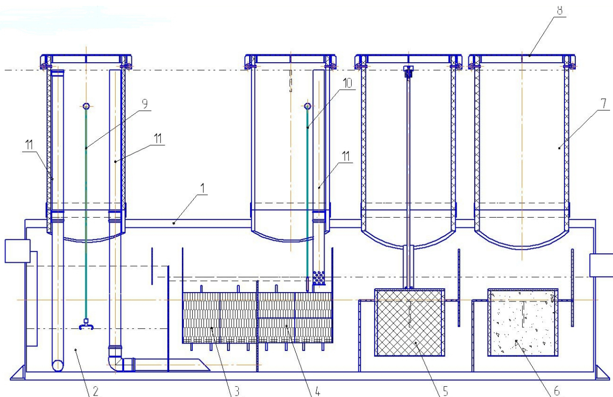
Рис. Пример песконефтеуловителя в сборе
