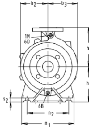
Etanorm C
